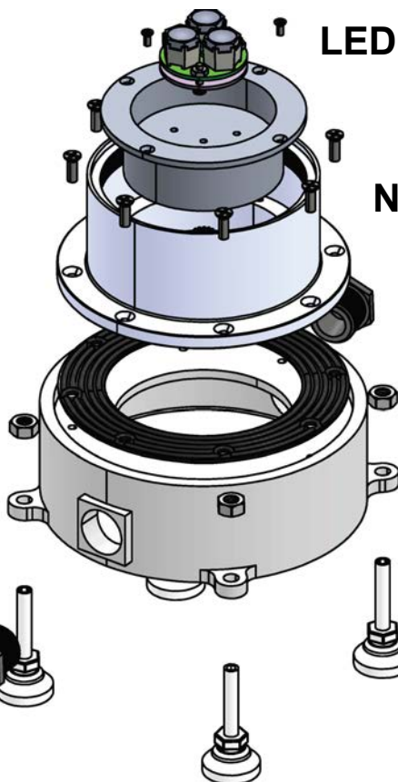
LEVELING STAND
