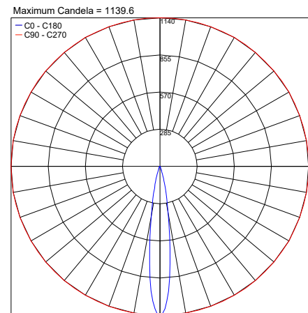
PHOTOMETRIC FILENAME : SPY MINI 30K 14°X20° - 43103.X.3.04.IES
