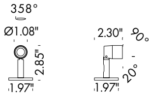
MINI FLOODLIGHT
