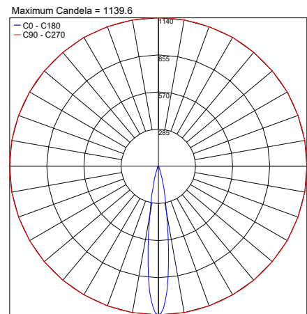
PHOTOMETRIC FILENAME : SPY MINI 30K 14°X20° - 43103.X.3.04.IES
