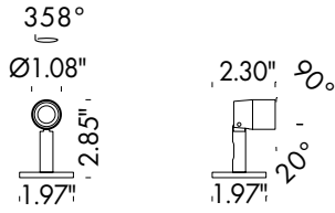
MINI FLOODLIGHT
