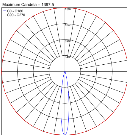
PHOTOMETRIC FILENAME : SPY MINI 30K 10° - 43103.X.3.01.IES
