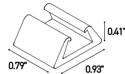
CLIP-S-14x6.5.W Silicone Clip
