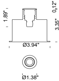
FLEA MINI Recessed Round Trim
