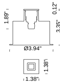
FLEA MINI Recessed Square Trim
