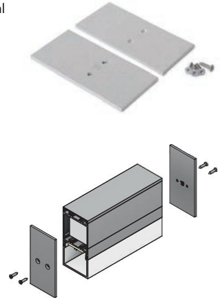
end cap VARIO30-19-E9 metal
